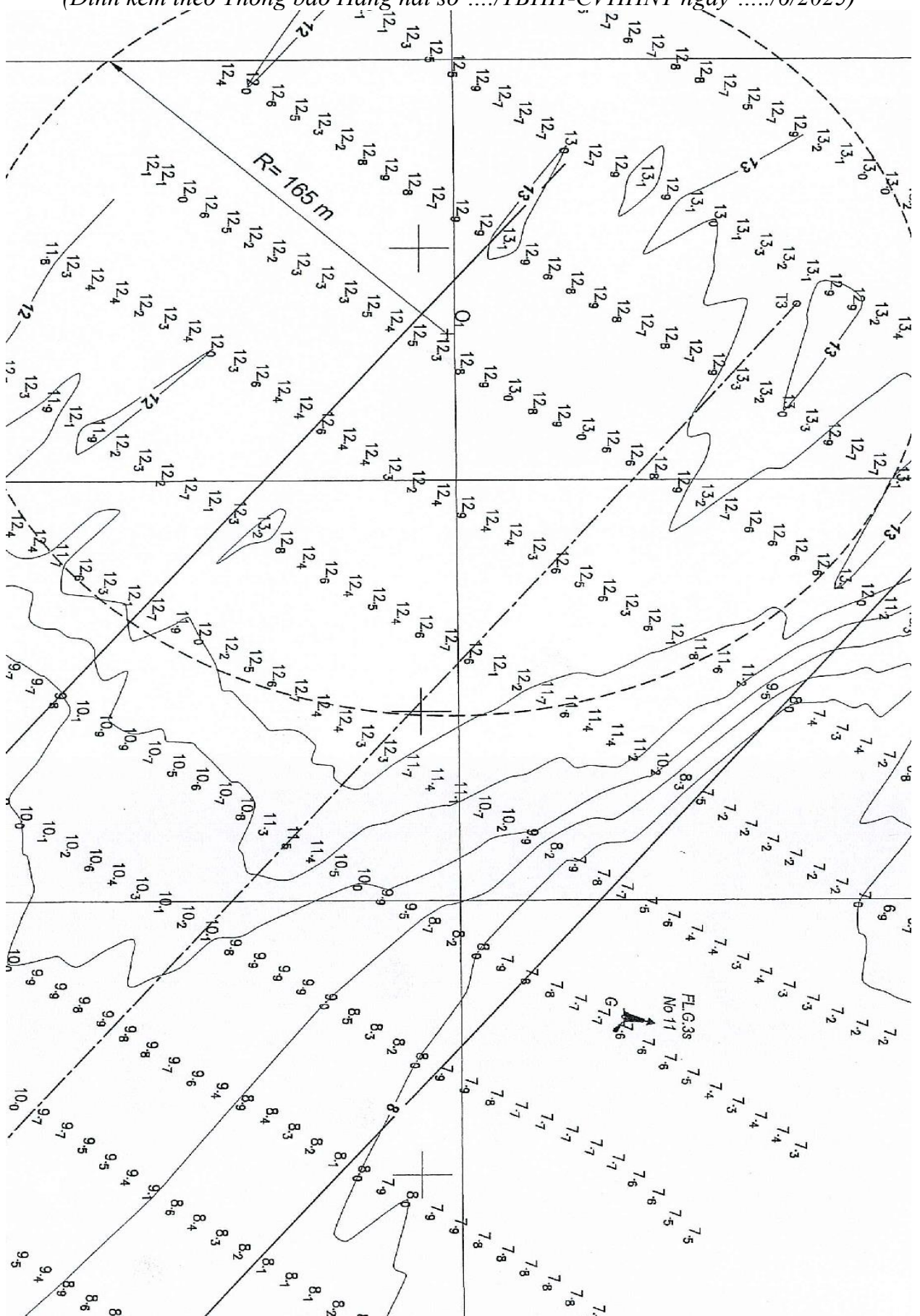
Hình ảnh 02: Trích dẫn bình đồ độ sâu ký hiệu BN_2505_08, tỷ lệ 1/2000 (Đính kèm theo Thông báo Hàng hải số ..../TBHH-CVHHNT ngày ...../6/2025)
